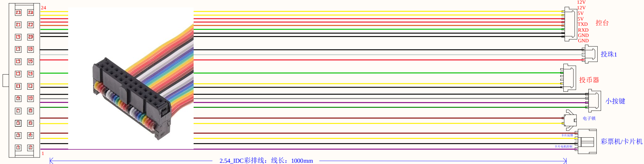
A1:弹界球盘线束图
